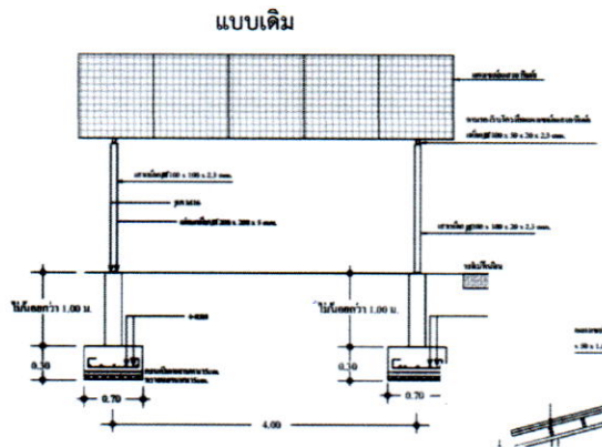
จุดที่ ๒ แก่ฐานรากคอนกรีตรองรับแผงโซล่าเซลล์แสงอาทิตย์
