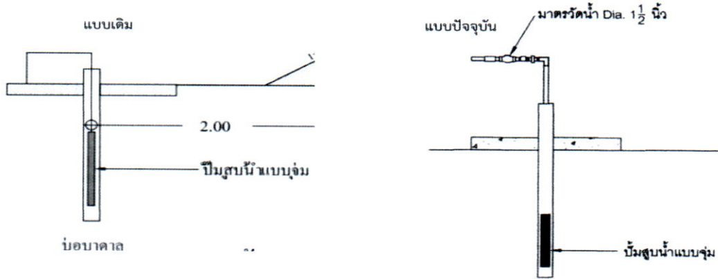
จุดที่ ๓ แก่ลานคอนกรีตรอบปากบ่อ/และเพิ่มมาตรวัดน้ำ
