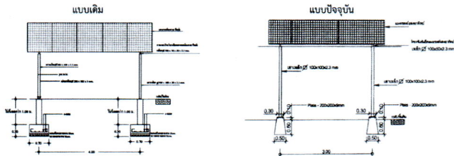
จุดที่ ๒ ฐานรากคอนกรีตรองรับแผงโซลาร์เซลล์แสงอาทิตย์
